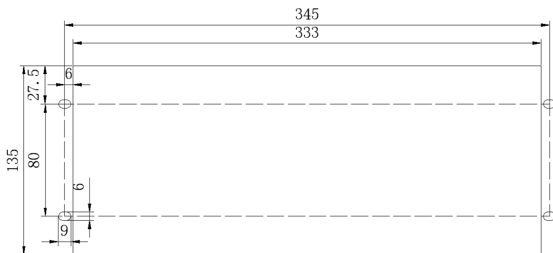
FYXH-16. A1 开孔尺寸图
